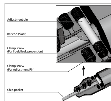
Fig. 3: Fixed bar
